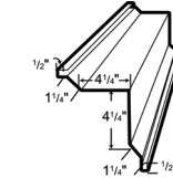
LG 125 9 1/4" DOOR JAMB
