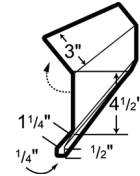
LG 130 SLIDING DOOR DRIP CAP
