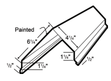
LG 126 DOOR POST TRIM*
